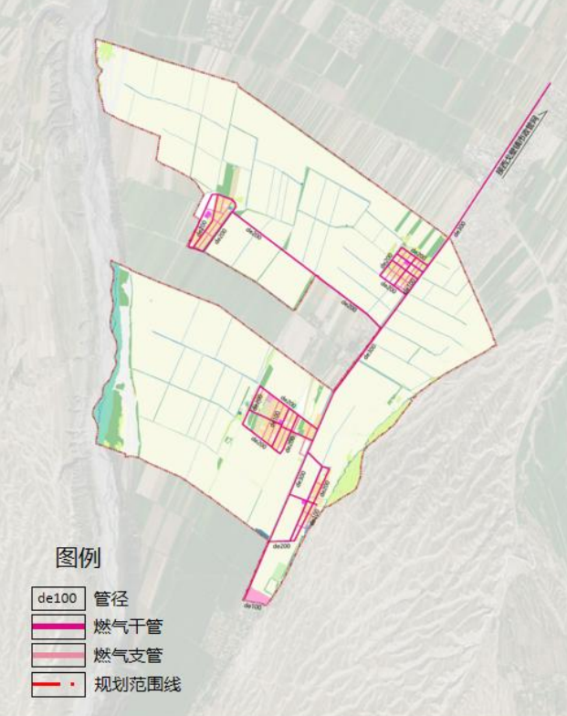
燃气工程规划
