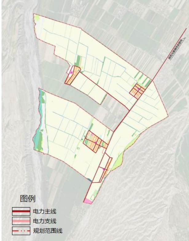
电力工程规划
