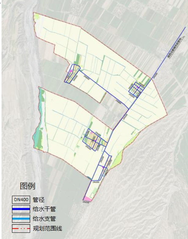
给水工程规划
